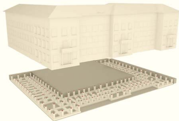
Figura 1: Schema intervento inserimento isolatori sismici corpo principale
